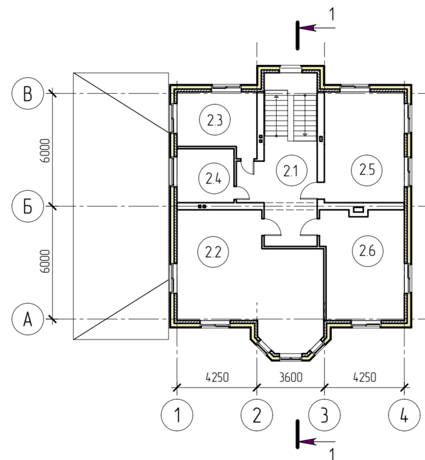
Общий вид
