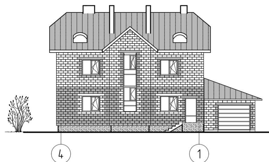
Фасад А-В
