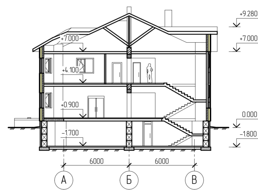
Разрез 1-1
