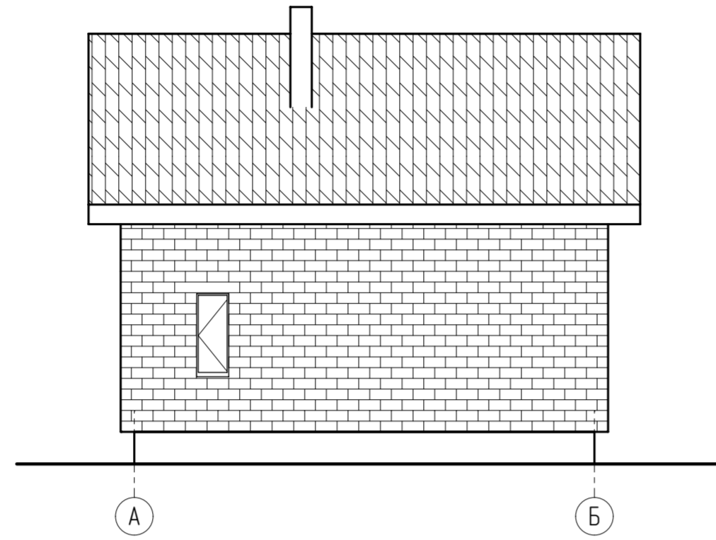
Фасад А-Б
