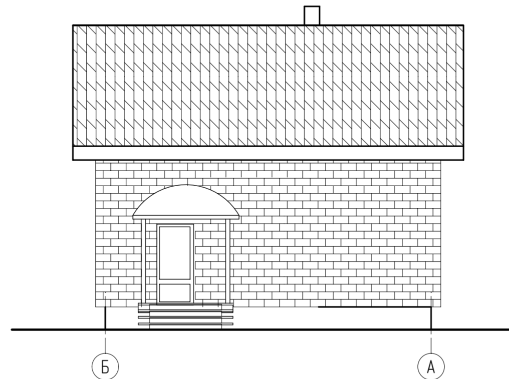
Фасад Б-А
