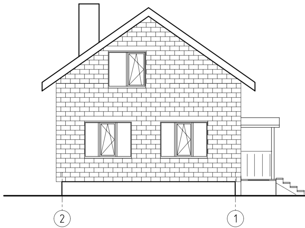
Фасад 2-1
